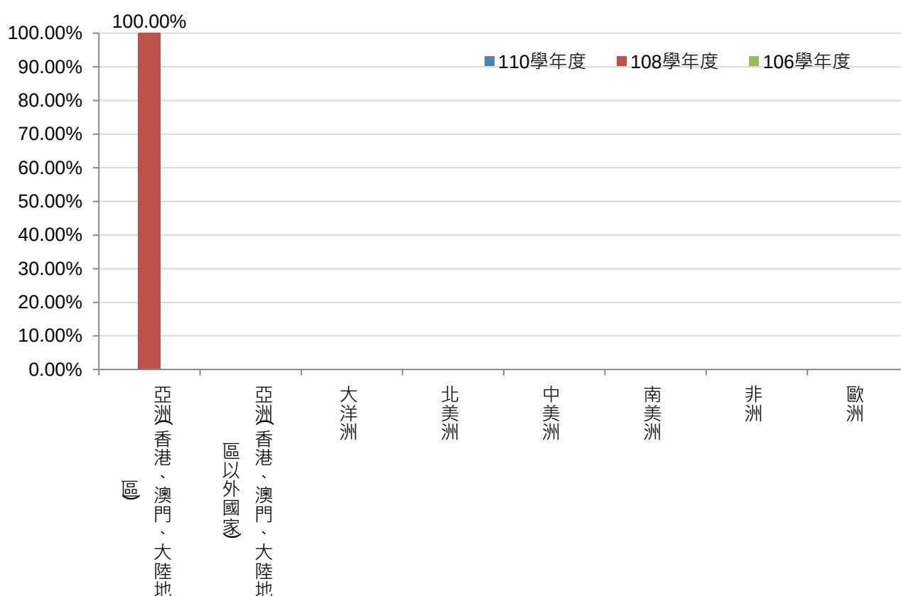
圖 57 境外就業地區分布圖(博士班)
