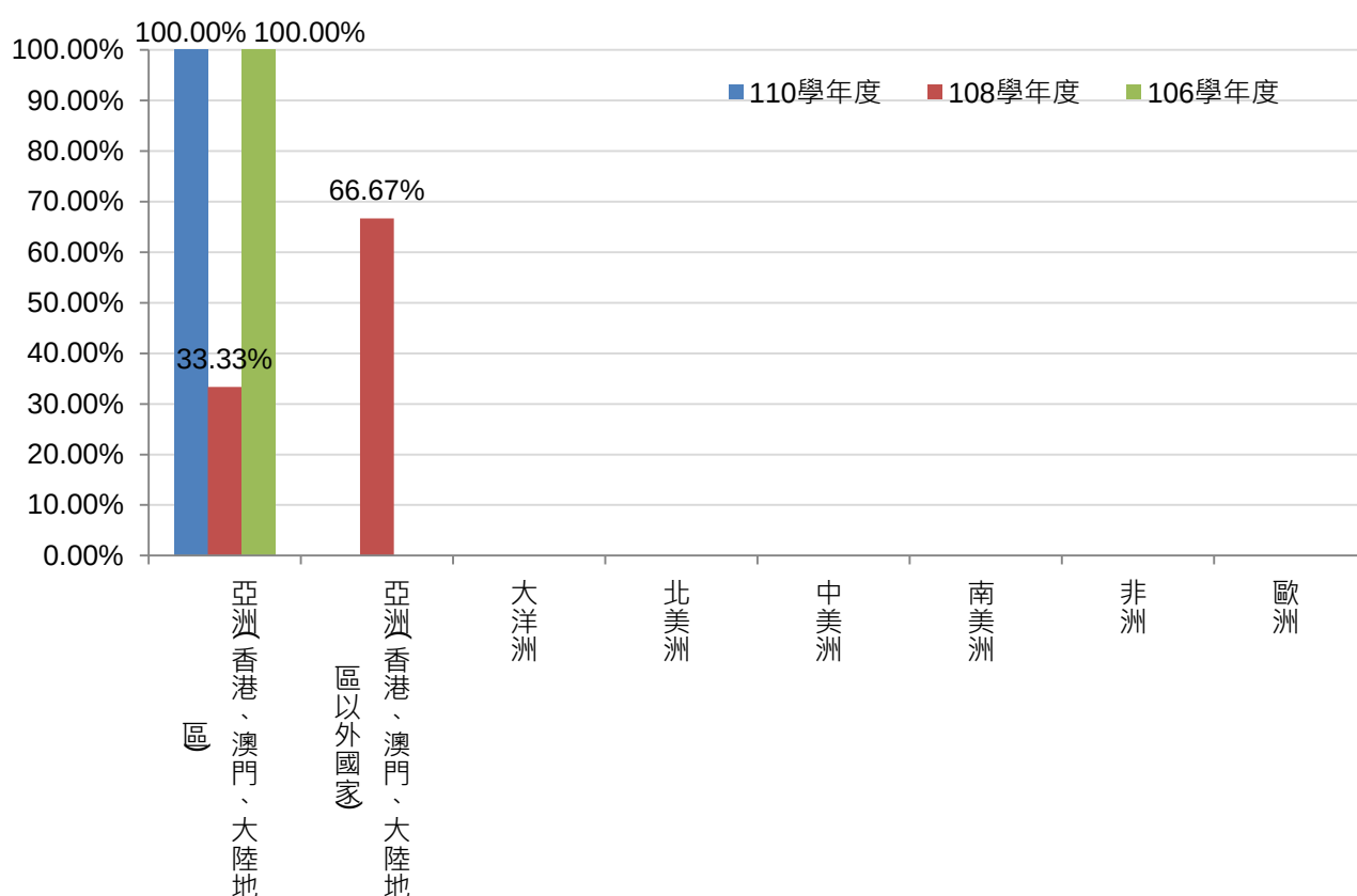
圖 30 境外就業地區分布圖(碩士班)
